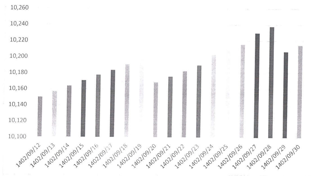
نرخ ابطال
